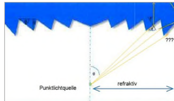
refraktive Struktur
