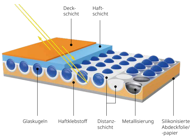
Aufbau mit eingebetteten Glaskugeln Design A
